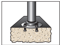
Poste para montaje en superficie (FGHPSM)
